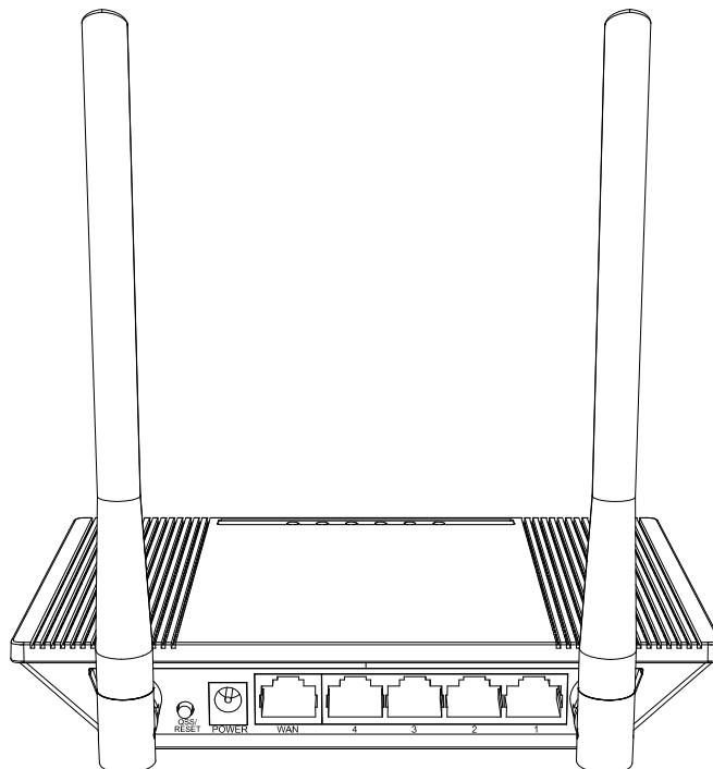
图 3-2 TL-WR847N 后面板示意图
