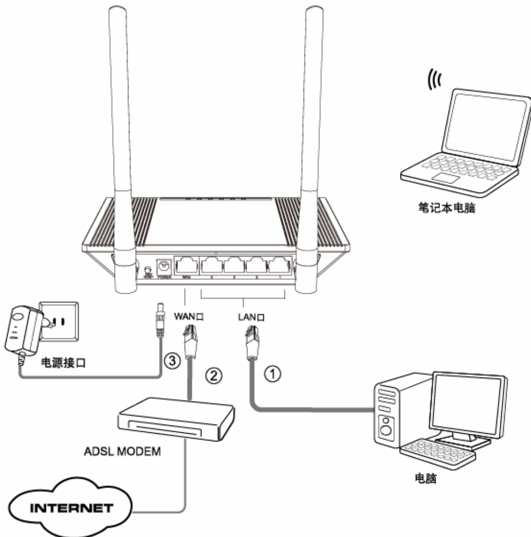
图 4-1 TL-WR847N 硬件安装示意图
